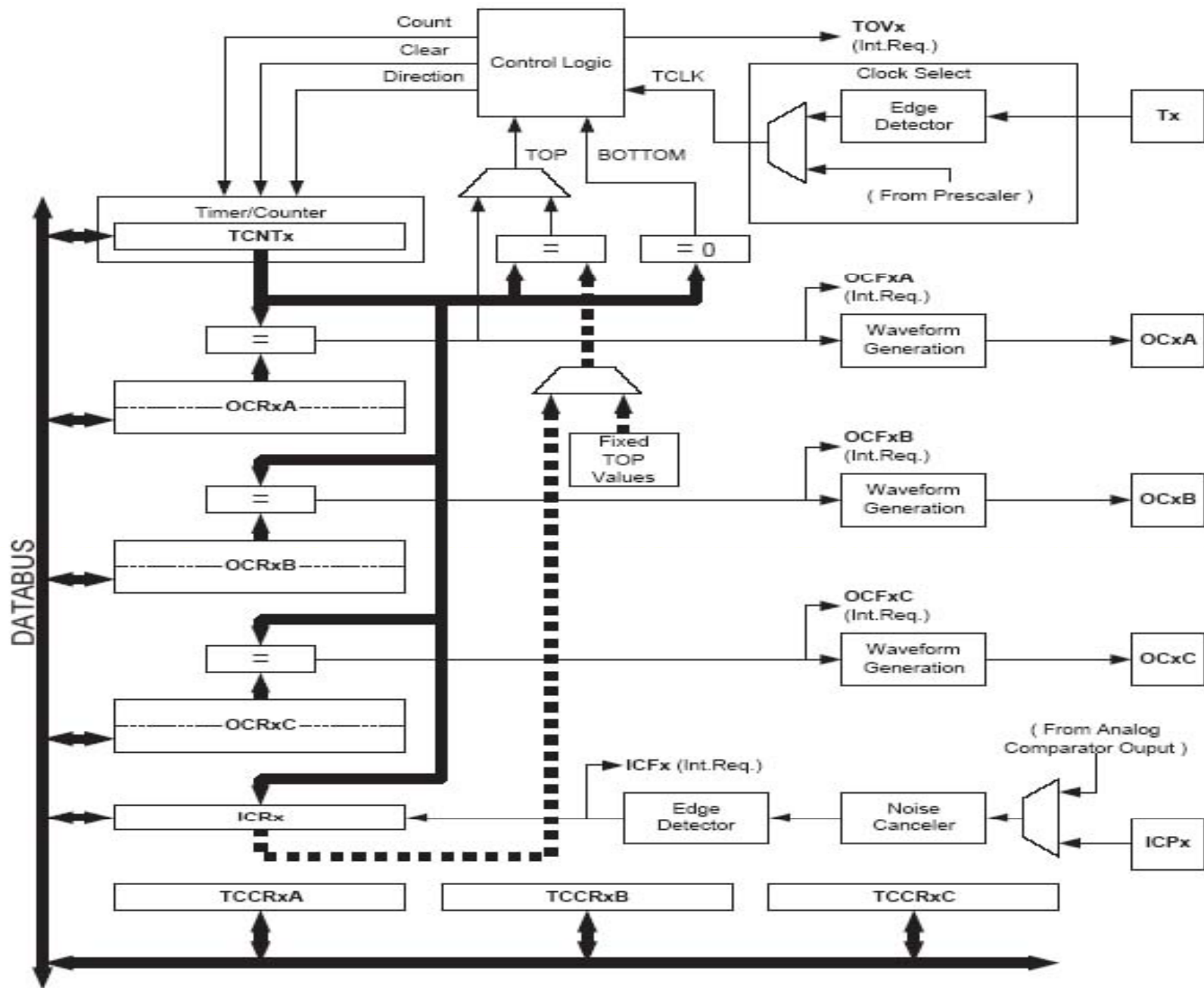
타이머/카운터 1의 블록도
