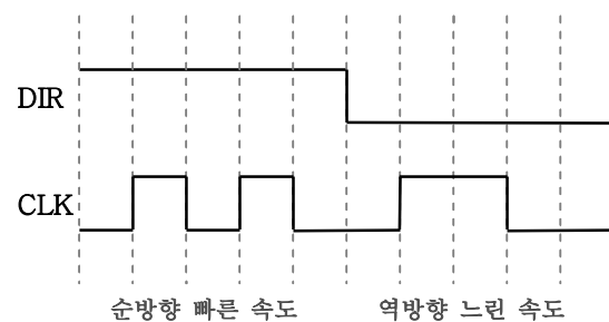
스테핑 모터 클럭 구동모듈 AM-MS2 입력 신호 : Dir(방향), CLK(속도) 신호
