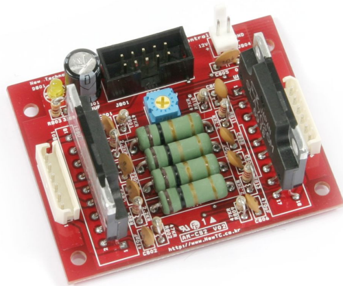
스테핑 모터 구동모듈 AM-CS2(P) 입력 신호 : A, /A, B, /B 각 상의 신호
