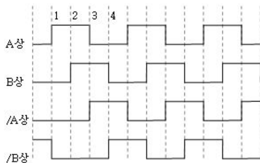
스테핑 모터 구동모듈 AM-CS2(P) 입력 신호 : A, /A, B, /B 각 상의 신호
