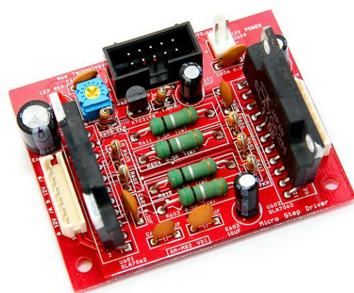
스테핑 모터 클럭 구동모듈 AM-MS2 입력 신호 : Dir(방향), CLK(속도) 신호
